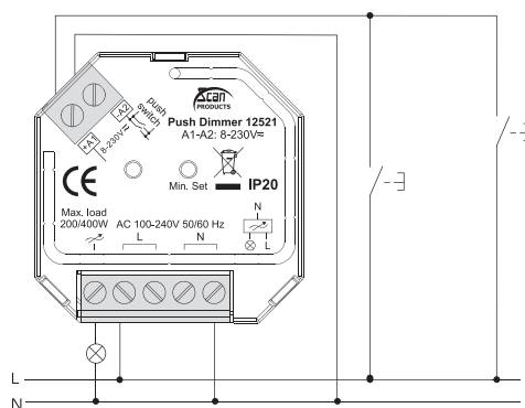
Ledningsdiagram
